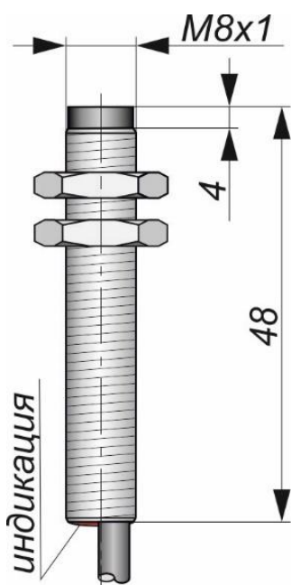
Габаритный чертеж
