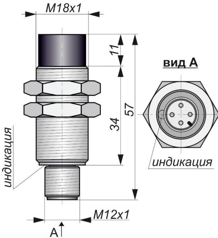
Габаритный чертеж
