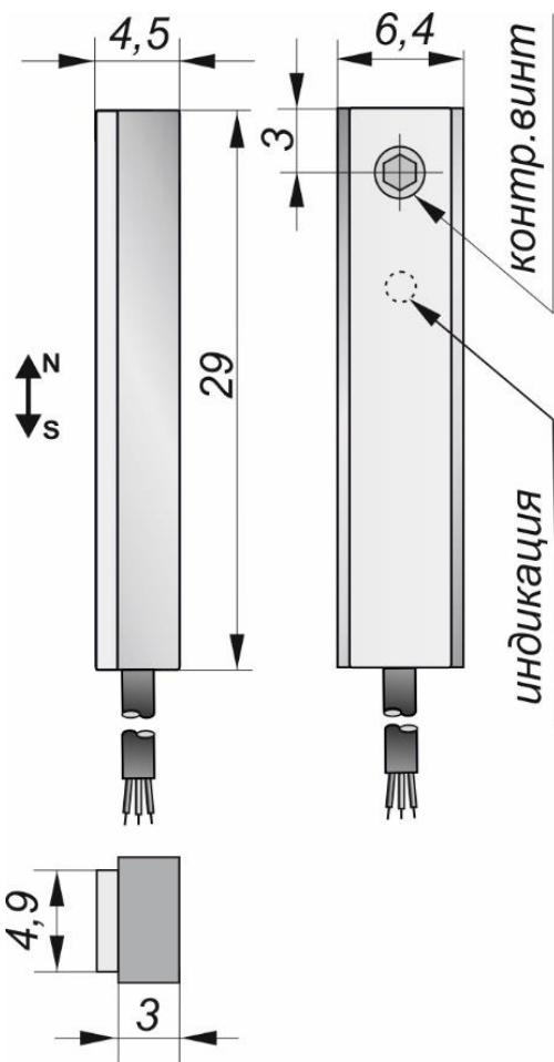
Габаритный чертеж
