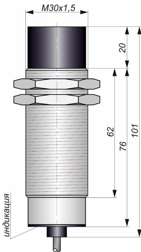
Габаритный чертеж
