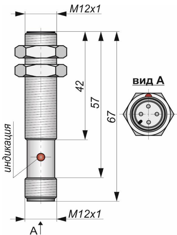
Габаритный чертеж
