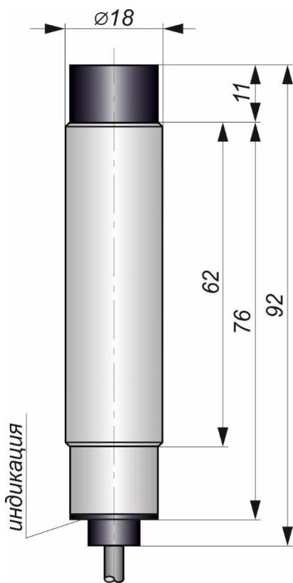
Габаритный чертеж
