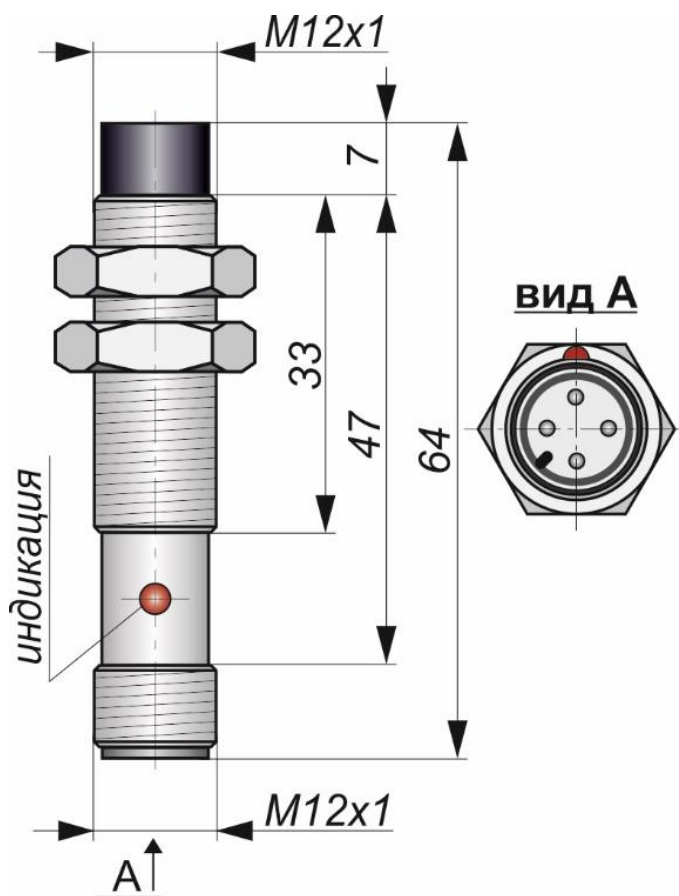
Габаритный чертеж
