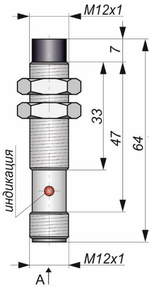
Габаритный чертеж
