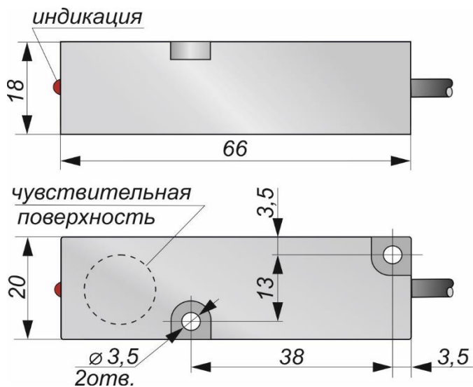
Габаритный чертеж
