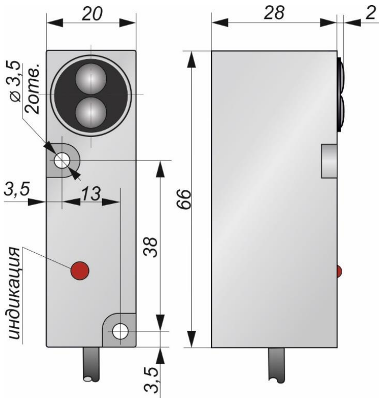
Габаритный чертеж
